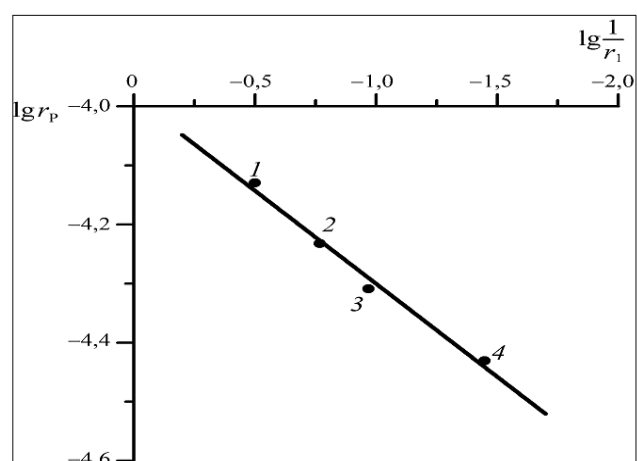
Рис. 4. Связь \lg r_p с \lg \frac{1}{r_1} винилкарбазолов в сополимеризации с винилбутиловым эфиром под действием SuCl_4 + CF_3COOH :
