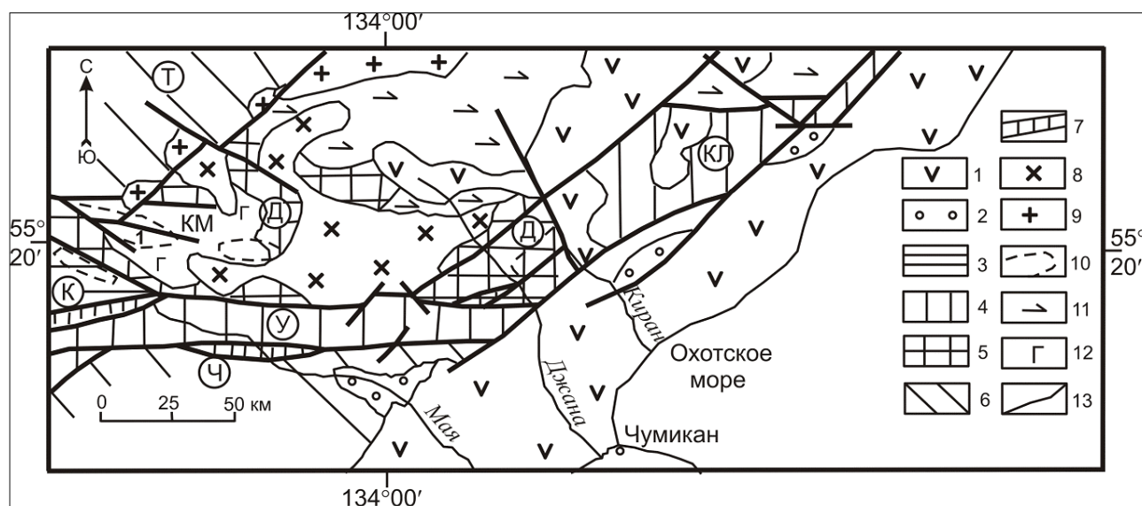
Рис. 1. Геолого-структурная схема юго-восточной окраины Алдано-Станового щита:
